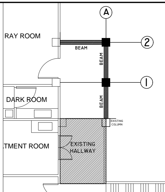
BEAM LAY-OUT
