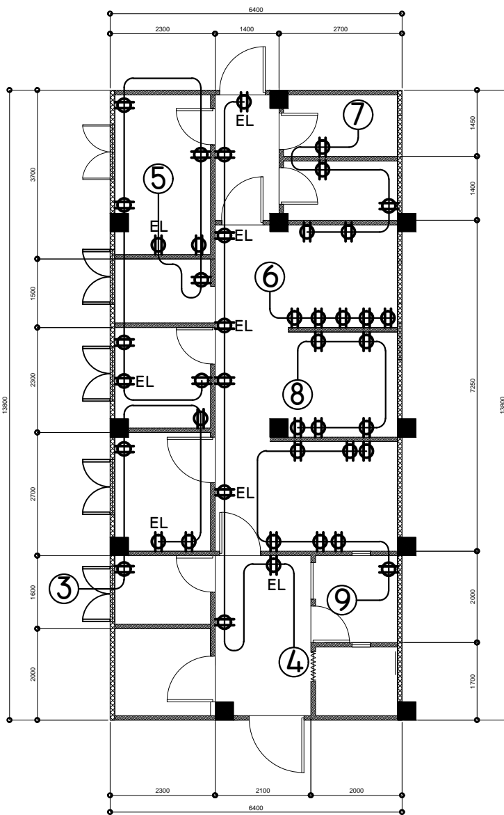
POWER LAY-OUT
